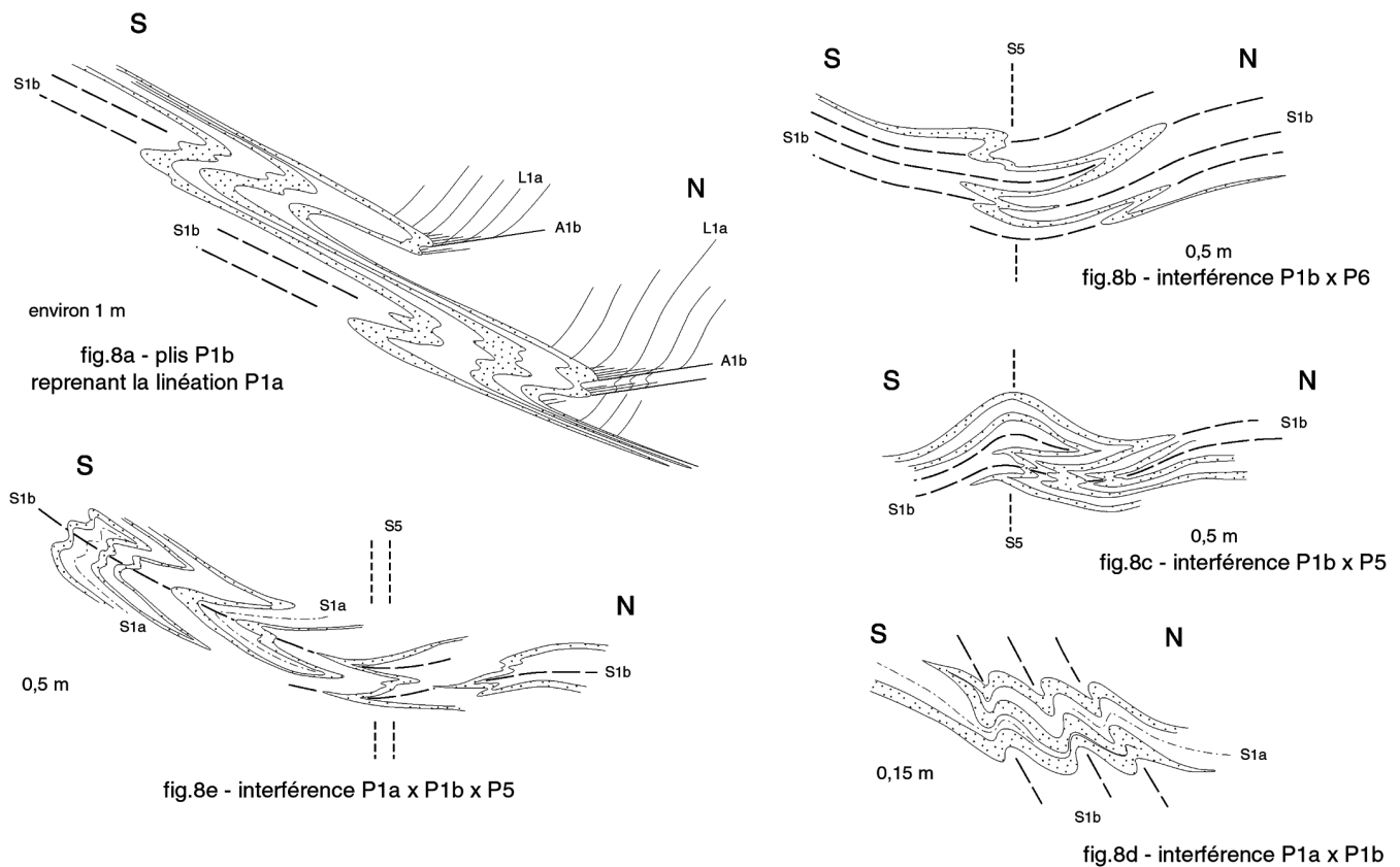
Fig. 8a-e.- La retombée nord de l'anticlinal du Caroux : affleurement de la forêt des Écrivains combattants. Les différents plis et leur interférence.
