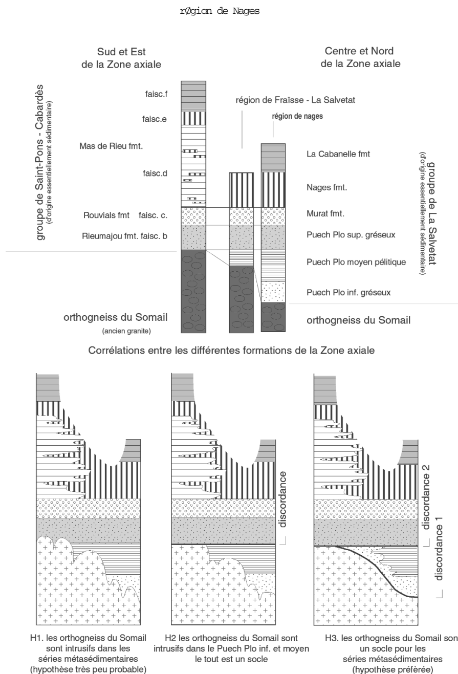
Fig. 16.- Corrélation entre les groupes de Saint-Pons – Cabardès et de La Salvetat. Différentes hypothèses quant aux rapports entre orthogneiss du Somail et formations métasédimentaires et à la définition d'un socle.
