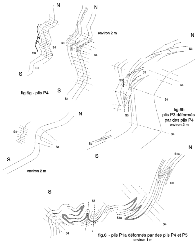
Fig. 6g-6i.- Coupe Prémian - Rouvials. 6h : p.c. 394 - 6g-i: 170 m au nord-ouest de ce point.
