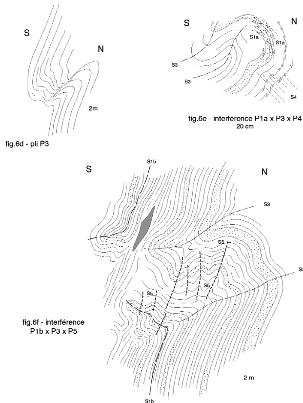
Fig. 6d-f.- Coupe Prémian - Rouvials. 6e : p.c. 394 - 6d-f : au « ball trap » 300 m au sud de ce point.
