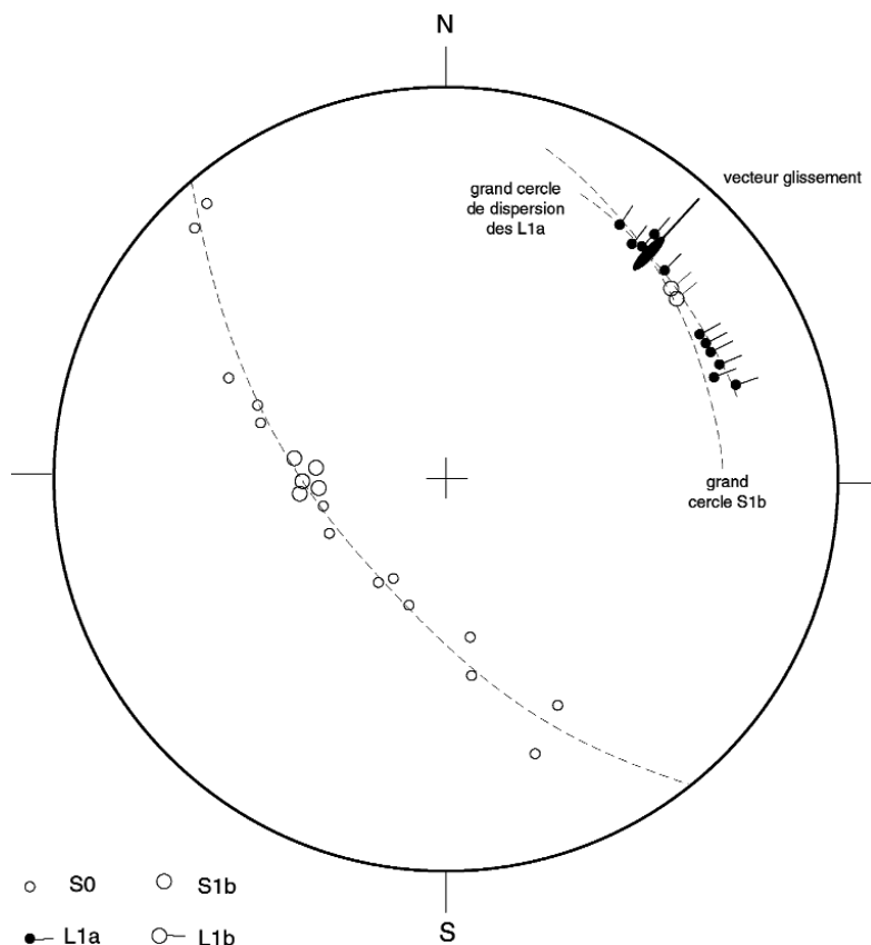
Fig. 15c.- Exemple de grande structure en plis couchés : la Serre de Nages. Diagramme La Tourelle.
