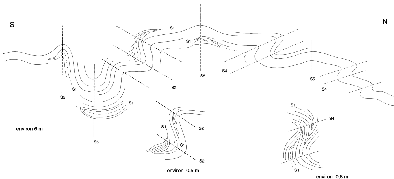
Fig. 11a.- La zone plate au centre du synclinal de Rosis : affleurement du col de Pierre Plantée. Plis superposés.
