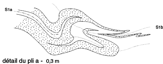
détail du pli a - 0,3 m
