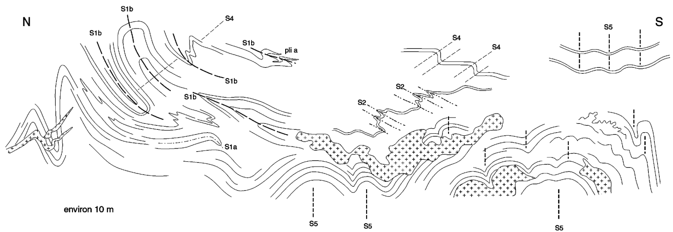
fig.7a - Mur de Cabrière
