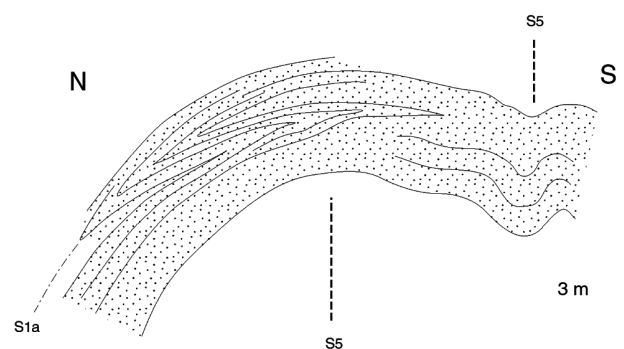
fig.7b - interférence P1a x P5
