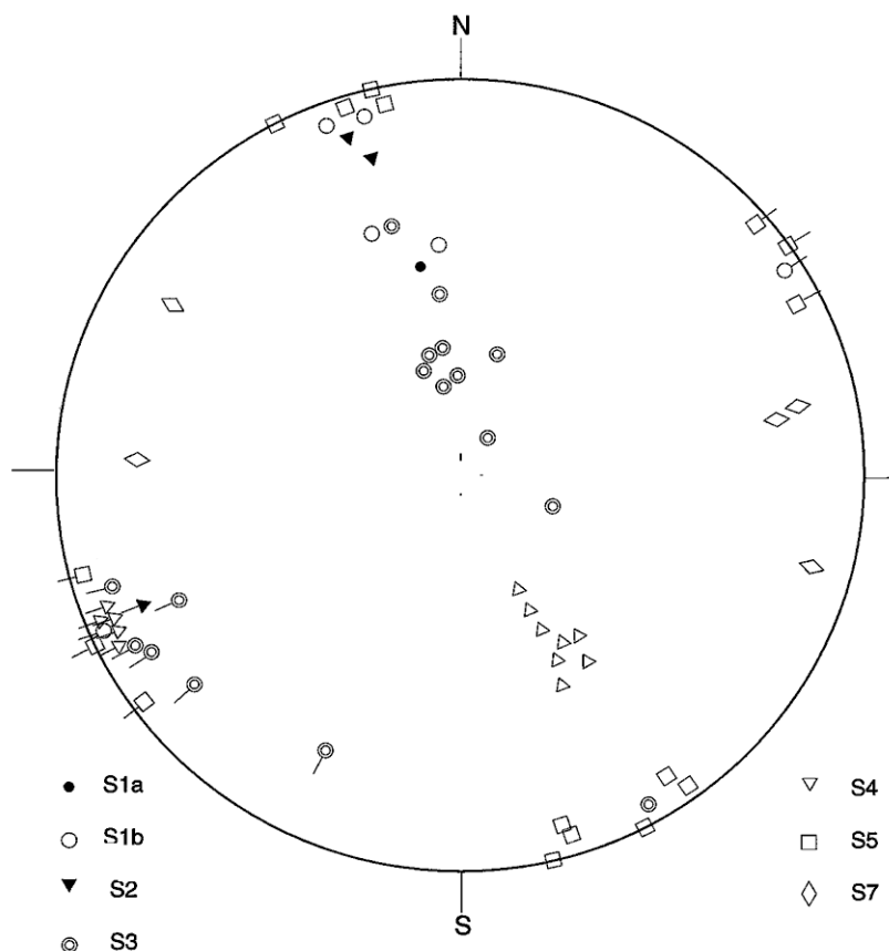
Fig. 6j.- Zone verticalisée au sud du massif de l'Agout : diagramme de Schmidt synthétique (projection sur l'hémisphère inférieure). Nous avons reporté sur ce diagramme les plis P3 déformés par P4 de la figure 5h ce qui fait que les plans S3 apparaissent beaucoup plus dispersés que les plans S1 et S2 ; la position la plus constante des plans S3 sur le flanc sud du massif de l'Agout est 85 S 20, là où sont concentrés la majorité des S3 sur le diagramme.
