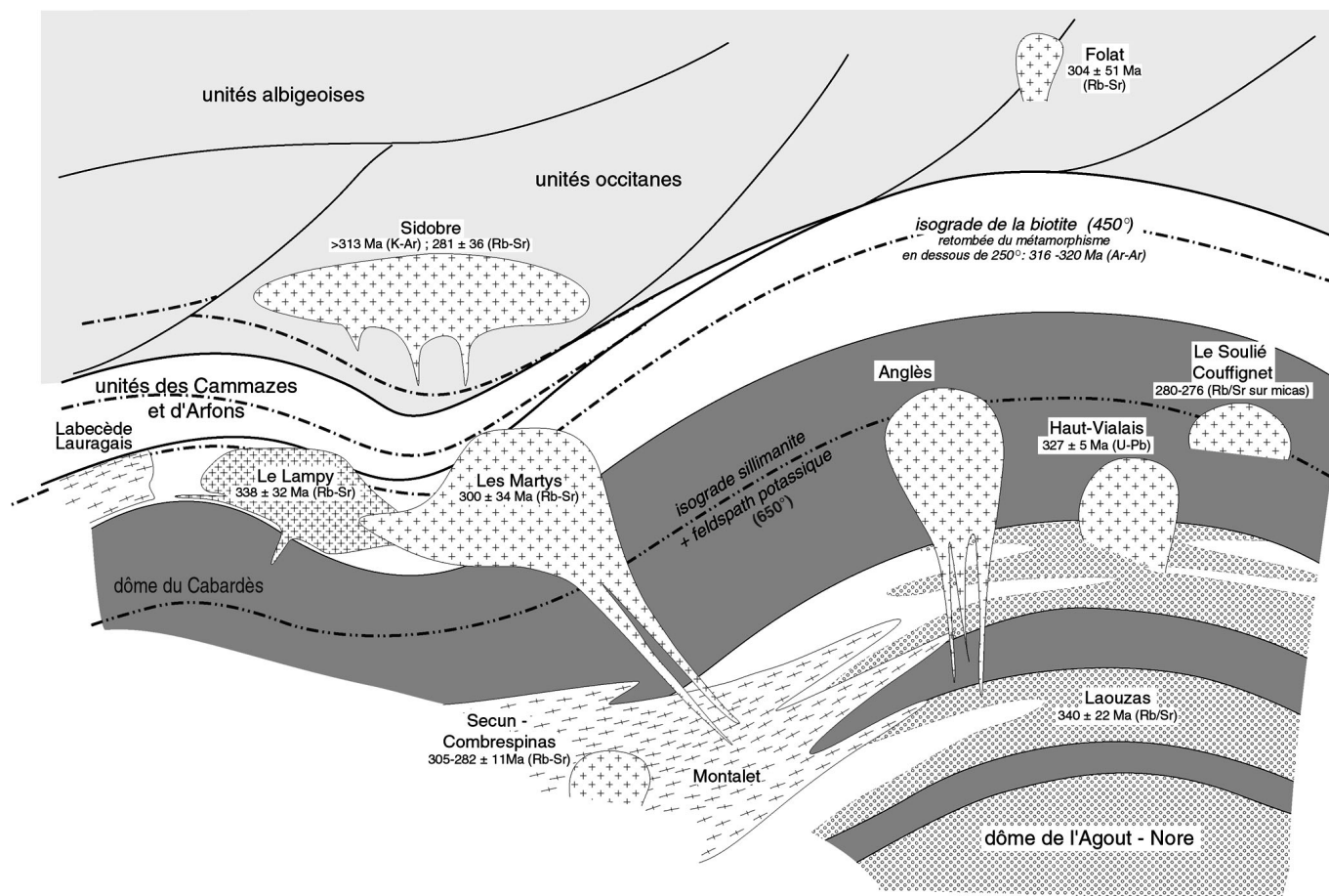
Fig. 23.- Niveau de mise en place des différents massifs granitiques de Montagne noire en fonction :
