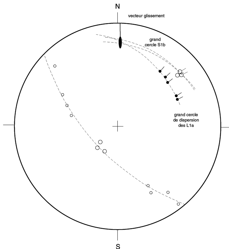
Fig. 15d.- Exemple de grande structure en plis couchés : la Serre de Nages. Diagramme Les Rieules.
