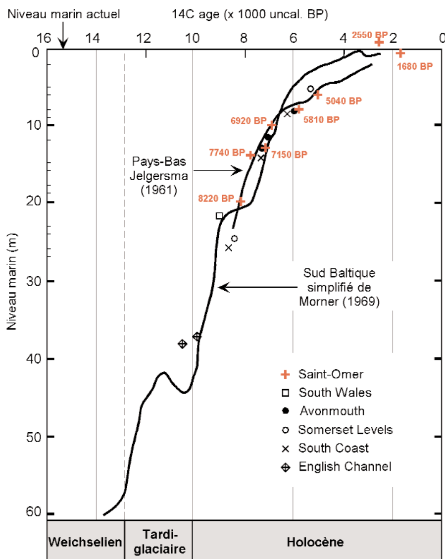
Fig. 11 - Remontée du niveau marin lors de la transgression tardiglaciaire/holocène (d'après Jelgersma, 1961 ; Mörner, 1969 ; in Hutchinson, 1992). Les dates radiocarbones sont non calibrées.
