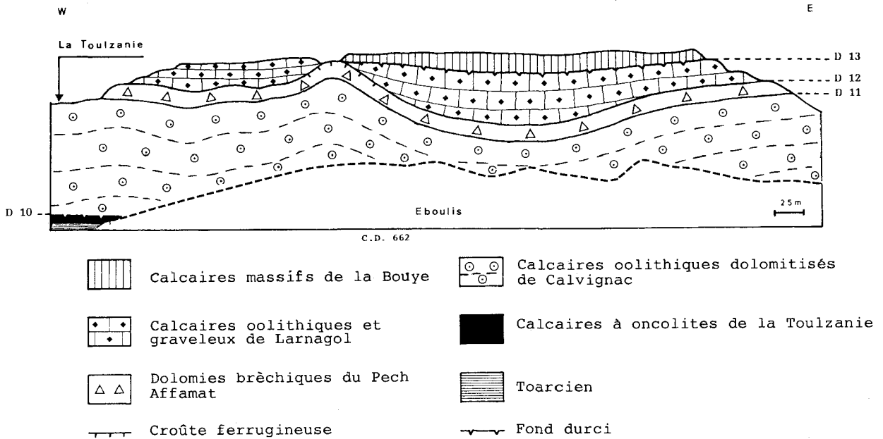
Fig. 5. - Les discontinuités bajociennes à la Toulzanie et la surface de discordance de la discontinuité D12.
