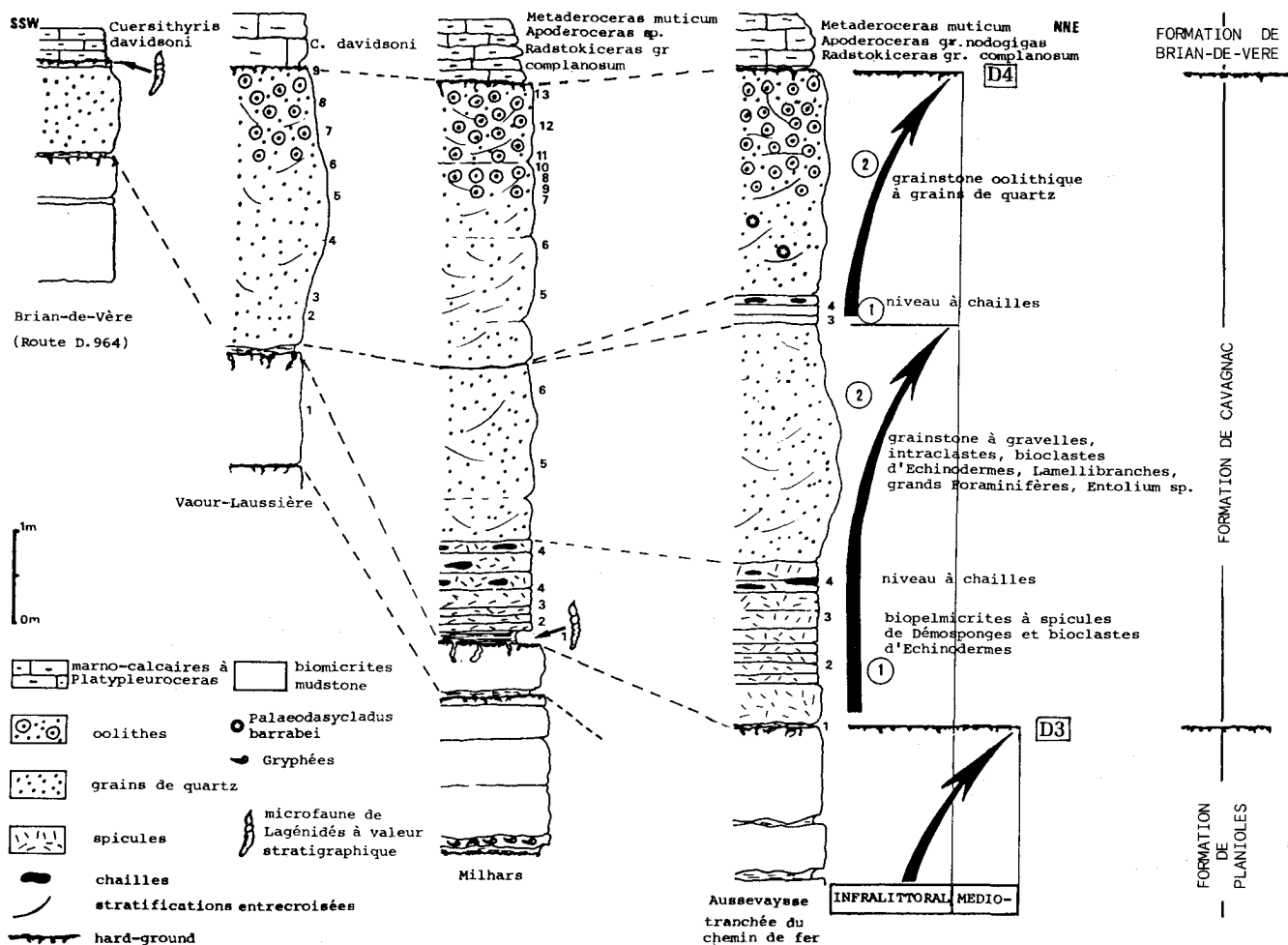
Fig. 12. - Coupes de la formation de Cavagnac dans la région de la Grésigne, montrant le dispositif en onlap au-dessus de la discontinuité D3.
