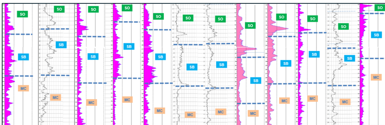
Figure 9 – Compilation d'extraits de diagraphies de radioactivité naturelle (gamma-ray) centrés sur les Sables de Beauchamp (entre les tiretés bleus). Les diagraphies s'étalent sur une distance plurikilométrique avec une distance variable entre chaque diagraphie. GPE, Ligne 16.
