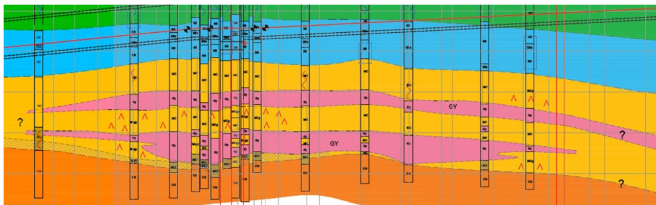
Figure 6 – Extrait (~1,6 km) d'un profil en long géologique du Grand Paris Express (L16) dans le secteur de Sevran où des lits de gypse d'épaisseur plurimétrique sont présents et préservés dans les Marnes et caillasses. La hauteur entre les lignes horizontales est de 10 m (échelle verticale = 10 x échelle horizontale).
