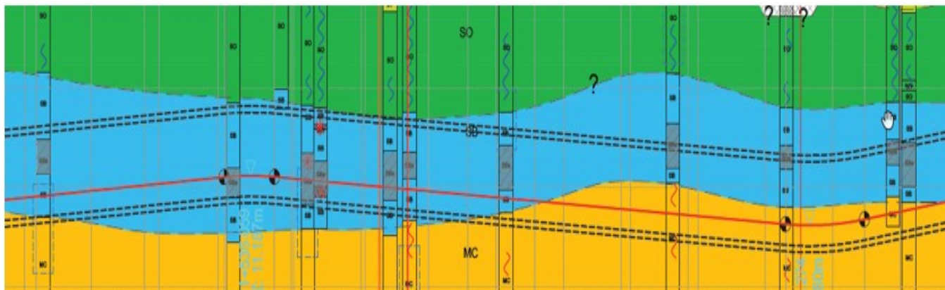
Figure 8 – Extrait d'un profil en long géologique d'un tronçon du GPE (L16, secteur St-Denis – Aubervilliers). Les sables de Beauchamp sont représentés en bleu et les niveaux argileux identifiés visuellement sur les carottes de sondages sont reportés en grisé sur les coupes de ces sondages. L'extrait couvre un linéaire d'environ 1,4 km, la couche des Sables de Beauchamp fait un peu plus de 10 m d'épaisseur.
