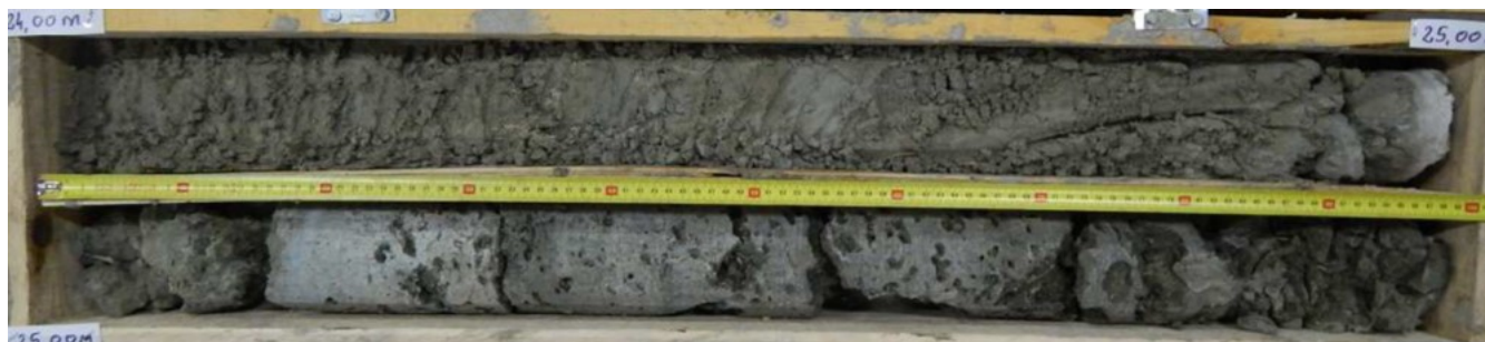
Figure 11 – Intercalation pluridécimétrique de calcaire dur et vacuolaire (carotte du bas) dans un encaissant sableux meuble. Sables de Beauchamp.
