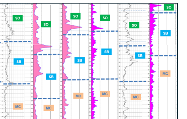
Figure 9 – Compilation d'extraits de diagraphies de radioactivité naturelle (gamma-ray) centrés sur les Sables de Beauchamp (entre les tiretés bleus). Les diagraphies s'étalent sur une distance plurikilométrique avec une distance variable entre chaque diagraphie. GPE, Ligne 16.
