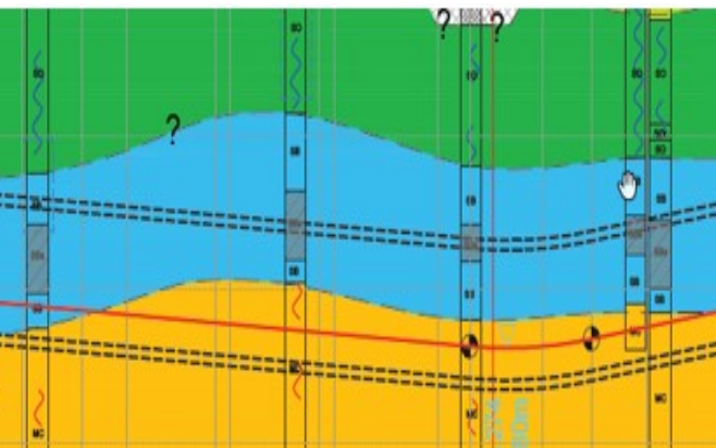
Figure 8 – Extrait d'un profil en long géologique d'un tronçon du GPE (L16, secteur St-Denis – Aubervilliers). Les sables de Beauchamp sont représentés en bleu et les niveaux argileux identifiés visuellement sur les carottes de sondages sont reportés en grisé sur les coupes de ces sondages. L'extrait couvre un linéaire d'environ 1,4 km, la couche des Sables de Beauchamp fait un peu plus de 10 m d'épaisseur.
