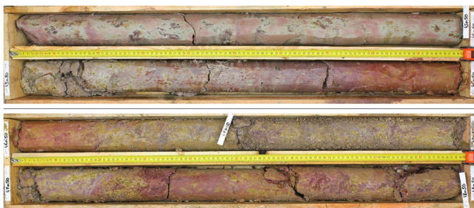
Figure 1 - Argile plastique : faciès bariolé typique. NB : sur toutes les photos de caisses de carottes présentées ci-après, celles-ci font 1 m de longueur.
