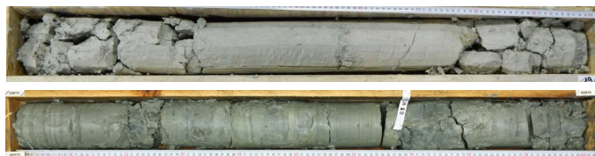
Figure 17 – Exemples de carottes de Marnes bleues d'Argenteuil (en bas) et de Marnes blanches de Pantin.
