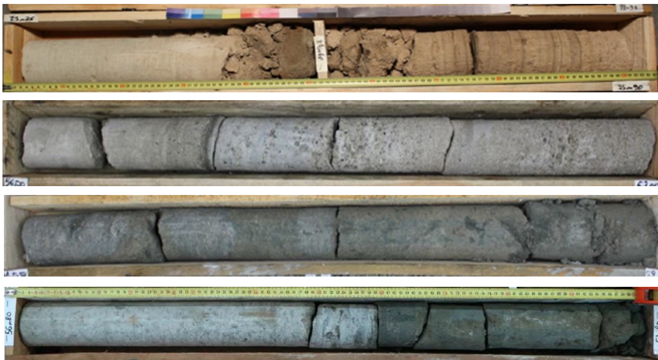
Figure 4 - Différents faciès ou bancs de la formation du Calcaire Grossier. De haut en bas : banc de calcaire clair, fin et dur (base du « Banc de Roche ») sur calcaire plus tendre et plus sombre ici lité (dolomitisé ?) ; calcaire gris rocheux à passées grossièrement fossilifère et vacuolaire ; calcaire irrégulièrement glauconieux et, en bas à droite, passée vert sombre plus tendre de composition probablement marneuse (banc vert possible).
