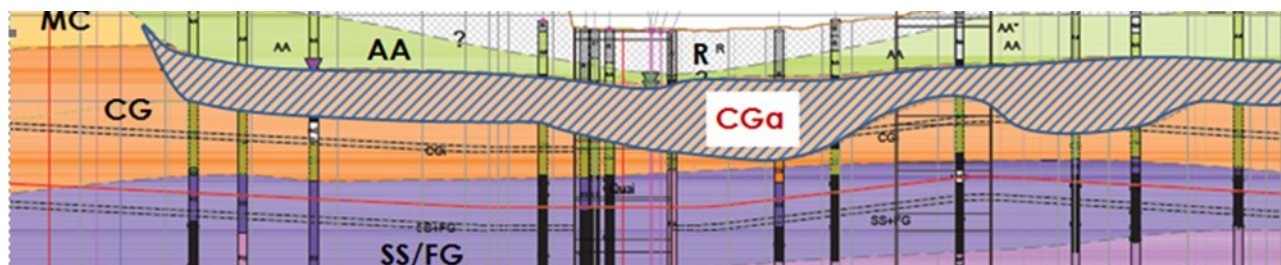
Figure 21 – Exemple d'intervalle altéré CGa (hachures) du Calcaire grossier en position superficielle. Extrait du profil géologique en long de la ligne 16 (secteur de la vallée de la Marne, près de Champigny). Longueur du profil = 1,5 km environ.
